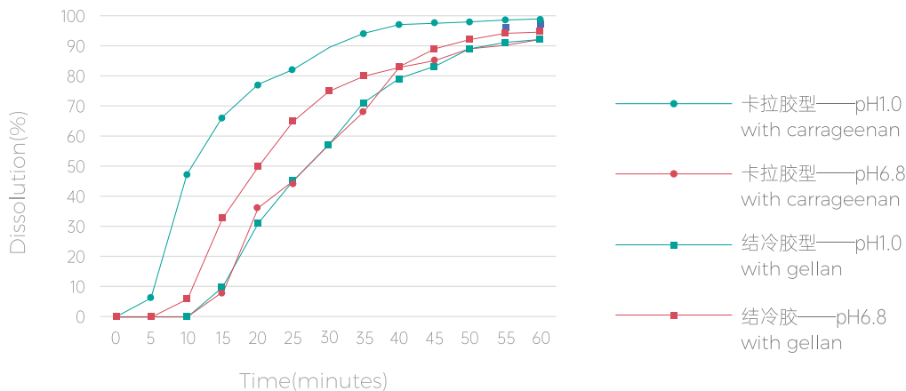
卡拉胶/结冷胶羟丙甲纤维素空心胶囊不同介质溶解速度 Empty Hypromellose Capsules with carrageenan/gellan gum dissolution performance
